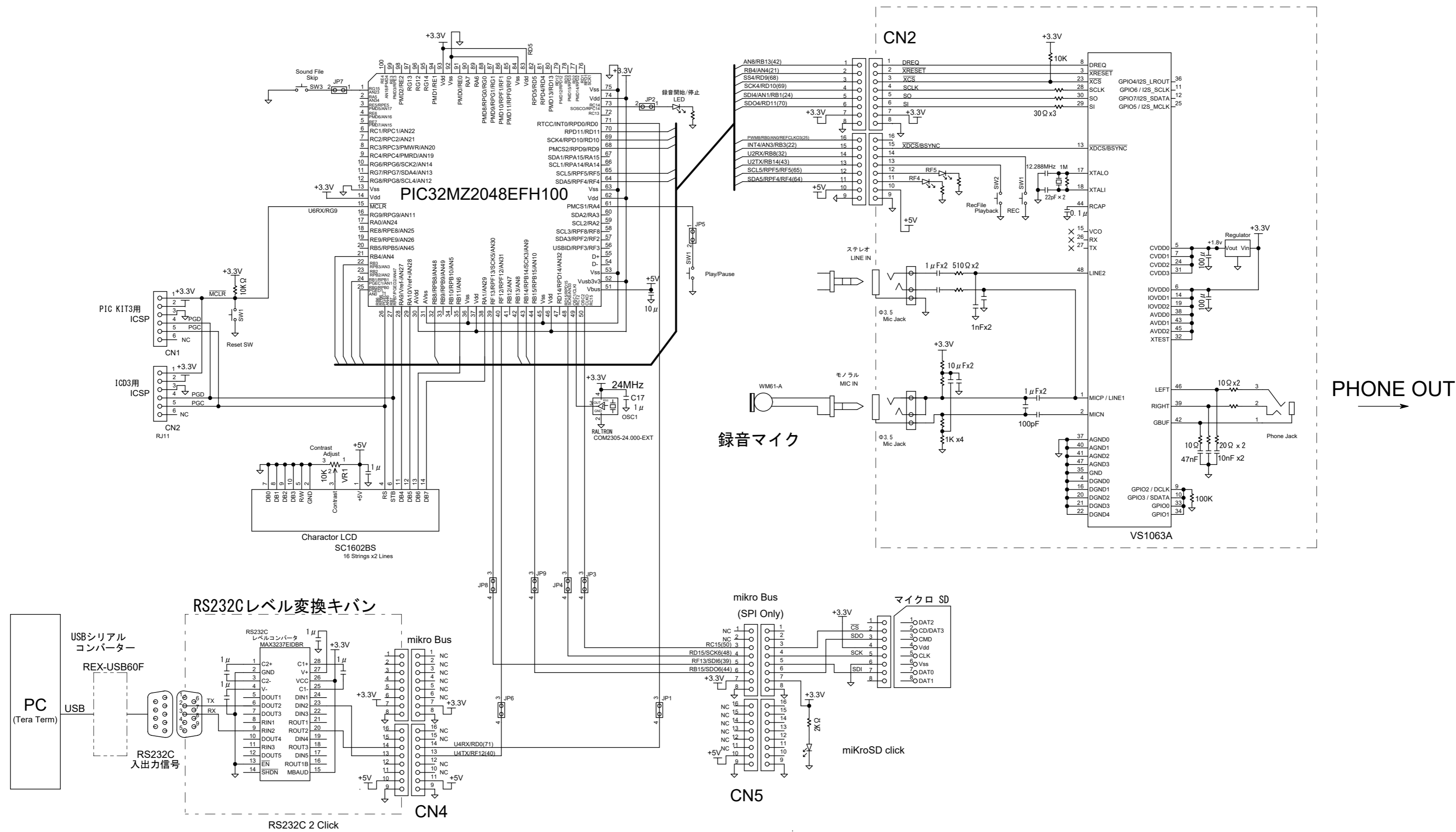
VS1063内臓エンコーダによる MP3ボイスレコーダー電気回路図
